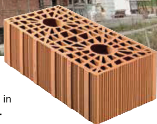
Il sistema Poroton Plan TS8 di DANESI coniuga i setti sottili al polistirene additivato con grafite, offrendo eccellenti performance termiche.
