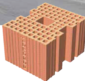
Blocco in laterizio P62/30 di CIS EDIL per murature portanti armate e antisismiche. Il complesso residenziale a Mirandola (nella foto) è stato realizzato con il blocco P62/30.
