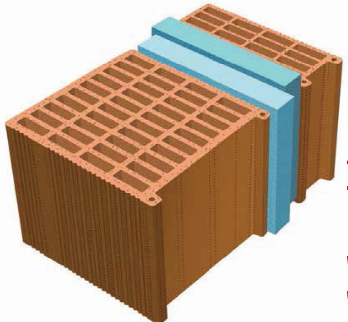
Normablok Blu8 42 Sismico , il blocco preassemblato impiegabile in tutte le zone sismiche per murature da 42 cm firmato P.C.L.
