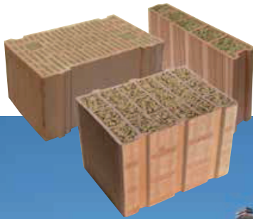
Brickwool System di LATERIZI ALAN METAURO è il sistema costruttivo ad alte prestazioni termoacustiche per murature portanti e di tamponamento.
